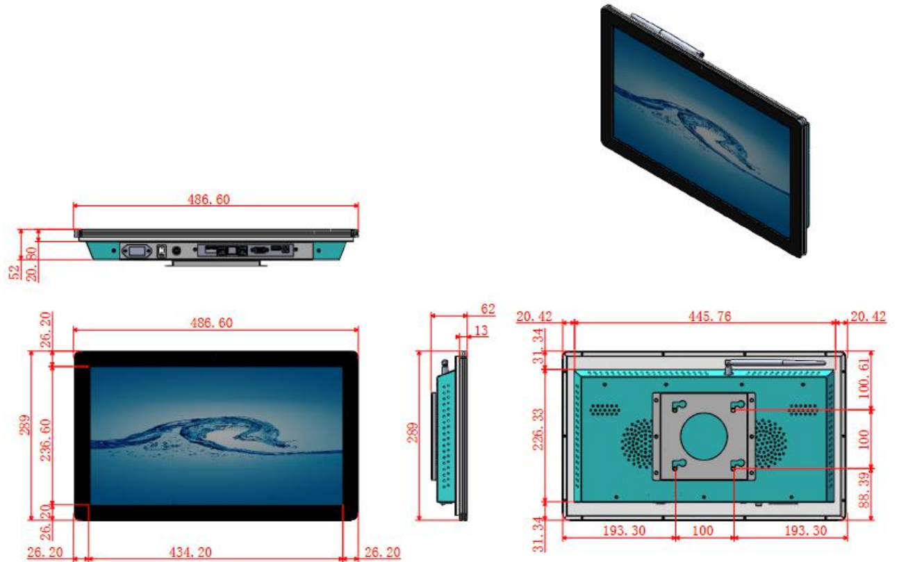
外观结构图:
